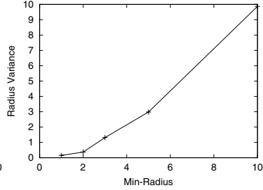
Fig. 16. Real Data(5)
