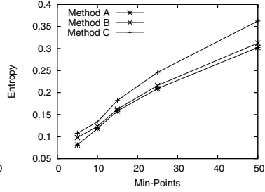
Fig. 10. Real Data(2)
