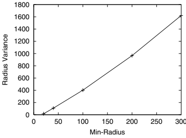
Fig. 15. Synthetic Data(5)
