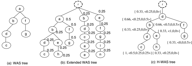
Fig. 2. Examples
