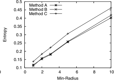
Fig. 8. Real Data(1)
