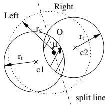
Fig. 5. Split
