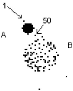
Fig. 5. A dataset
