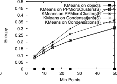
Fig. 12. Real Data(3)
